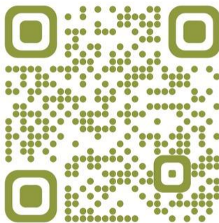
EDF DATABASE
